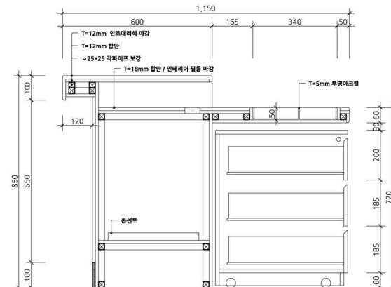
5 SECTION 1 T18mm합판 인테리어필름마감→HPM마감으로 변경
