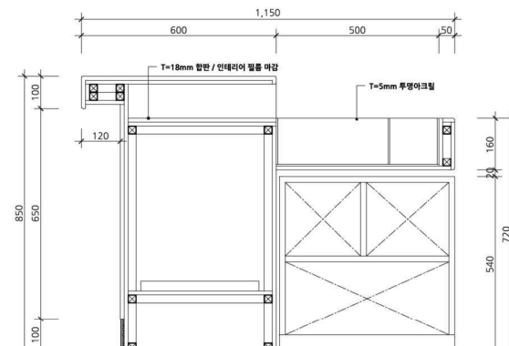
6 SECTION-2 T18mm합판 인테리어필름마감→HPM마감으로 변경
